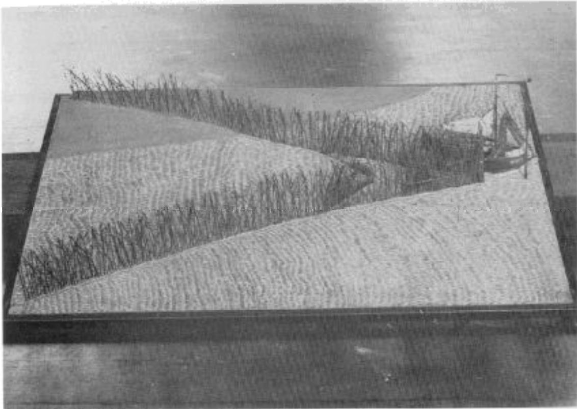
Het model van een weervisserij, aanwezig in het Gemeentemuseum te Bergen op Zoom. Het is laag water. De visserij is reeds klaar. De bovenste vleuk is drooggevallen, de fuik hangt in het want te drogen (foto van der Aa).
