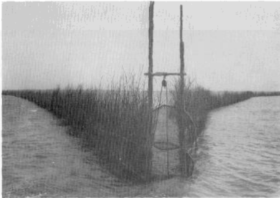
Weervisserij in de Oosterschelde. Het fuikgat, bij afwezigheid van de visser met een houten schroef gesloten, en de fuik die er tijdens het vissen wordt voor gezet (foto van der Aa).
